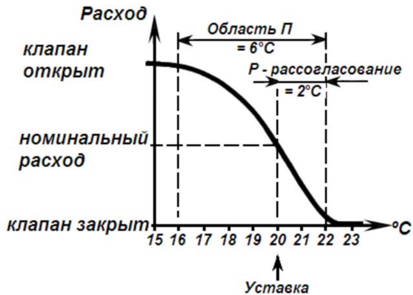
Рисунок 7.5 – Характеристика термостатического вентиля
