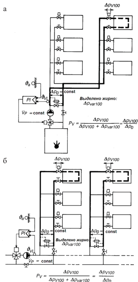
Рисунок 7.7 – Расчет авторитета клапана на примере 2-х систем
